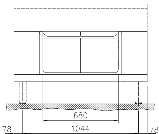
Zij aanzicht
