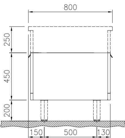
Zij aanzicht
